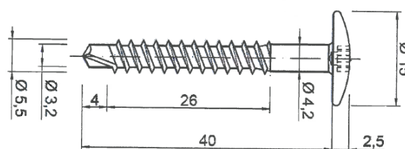
Viti autoforanti UNI-Screw per legno 5.5 x 40 mm per pannelli di spessore 8 mm
