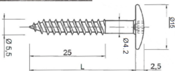
Vite UNI-Screw Standard per legno 5.5 x 35 mm per pannelli di spessore 8 mm
